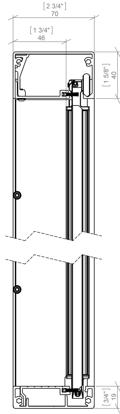
SECTION A-A
