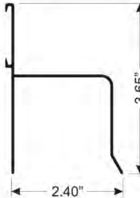
H Header Item: 757
