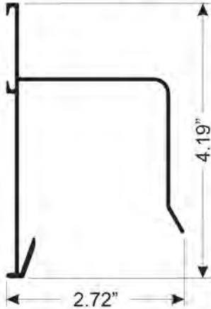
Ultra-H™ Header Item: 787
