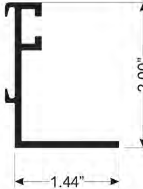
Ultra-LF™ Sill Item: 784A
